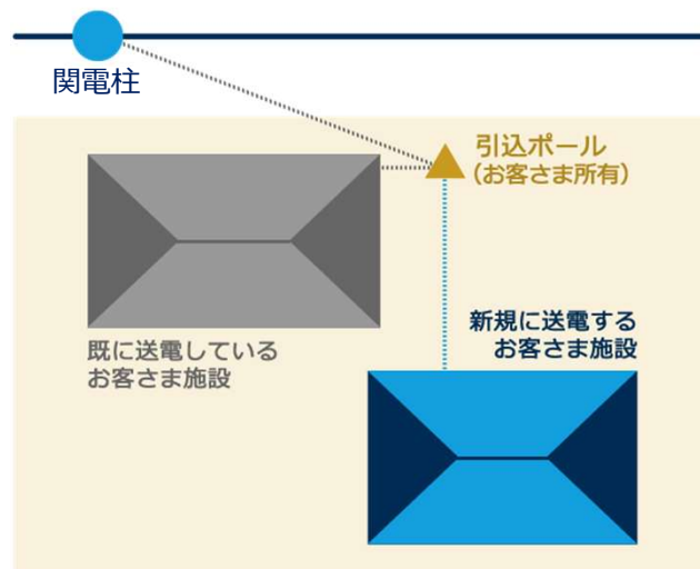
接続引込
